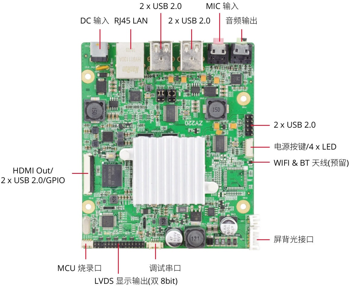
接口示意图：
